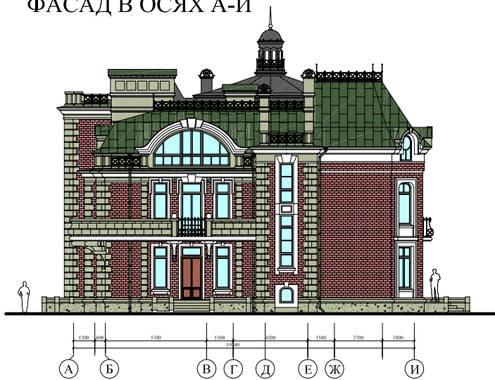
ФАСАД В ОСЯХ А-И
